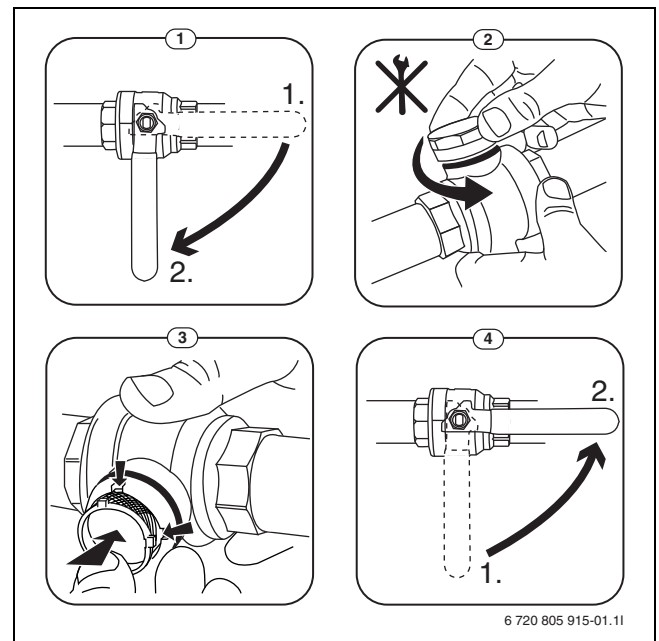
Rys. 8 Czyszczenie sitka
