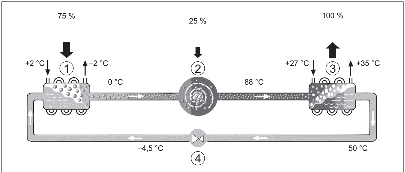
Rys. 2 Zasada działania obiegu czynnika chłodniczego w pompie ciepła
